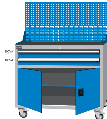
SPL-014DM 1020Lx572Wx825H+500
