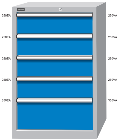
SPL-1023-17 1023Lx725Wx1450H
